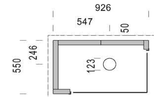
Position Zuluft Anschluss Deko 7R Uno
